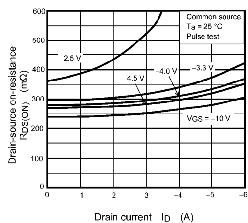
Fig. 9.4 R_{DS(ON)} - I_D
