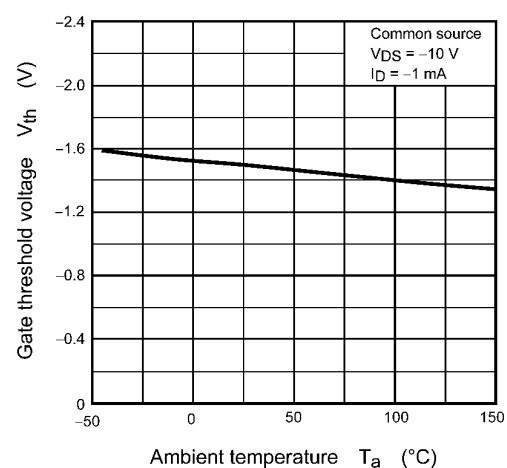
Fig. 9.6 V_{th} - T_a
