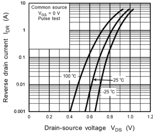
Fig. 9.7 I_{DR} - V_{DS}
