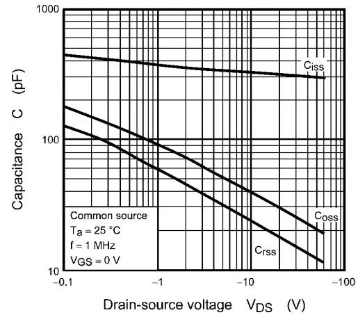
Fig. 9.8 C - V_{DS}
