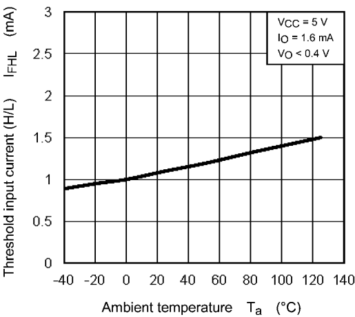
Fig. 12.2.7 I_{FHL} - T_a
