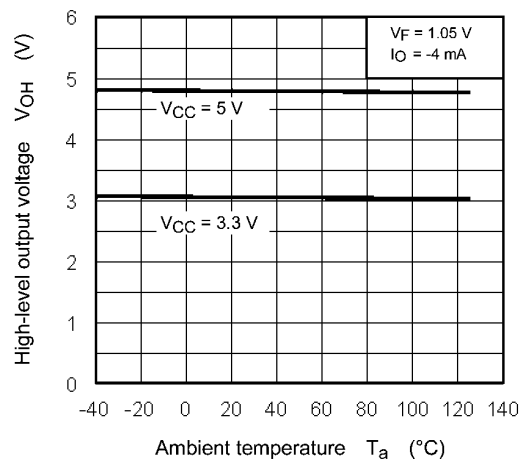
Fig. 12.2.4 V_{OH} - T_a
