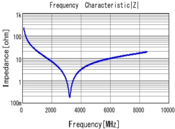
■ GCQ1555C1H7R0CB01 |Z| DC0V, 25degC
