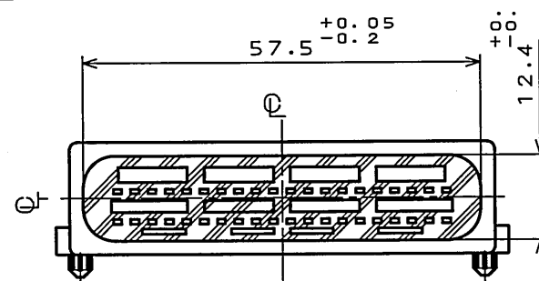
S E C T . B - B ( S C A L E 1 : 1 )
