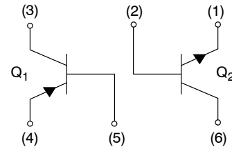
NST3946DP6T5G*
