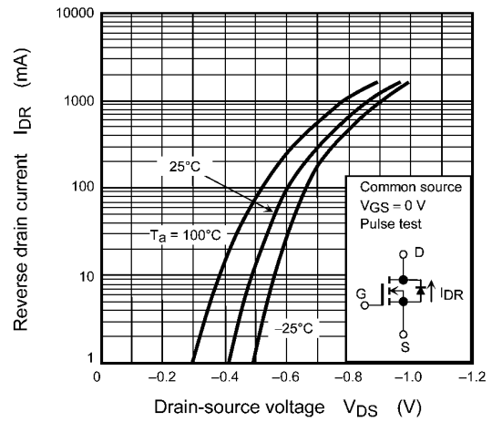
Fig. 7.8 I_{DR} - V_{DS}
