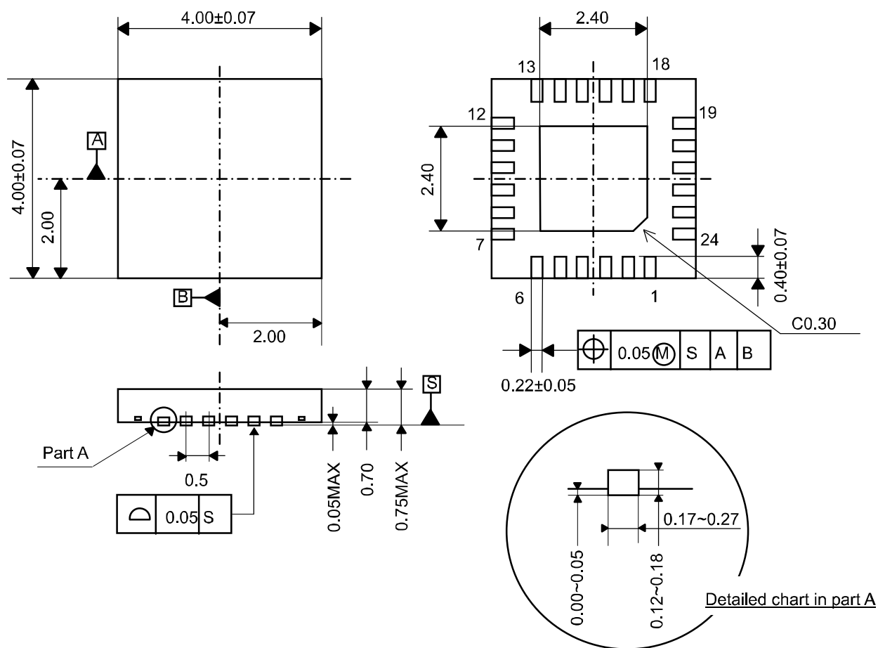
Fig. 15 Outer Dimensions
