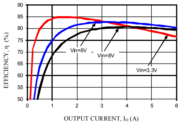
V_o = 0.6V
