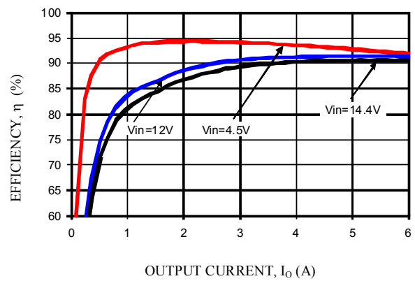
V_o = 2.5V
