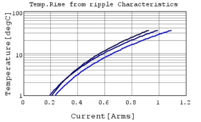
GRM1555C2A220JA01 Temp.rise 500MHz
