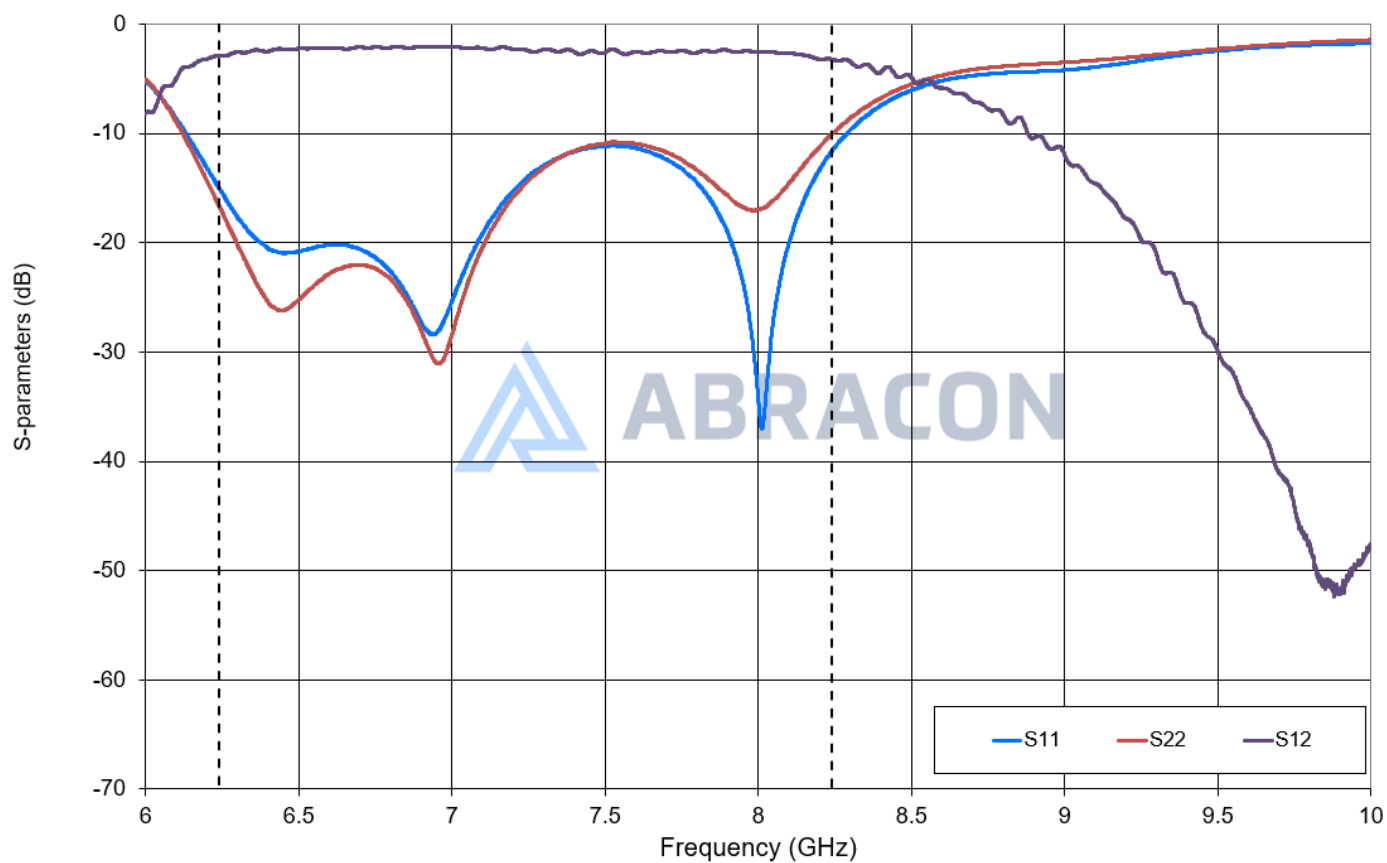
S-parameters
