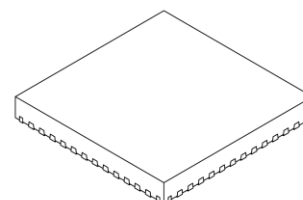
P-VQFN48-0707-0.50-004
