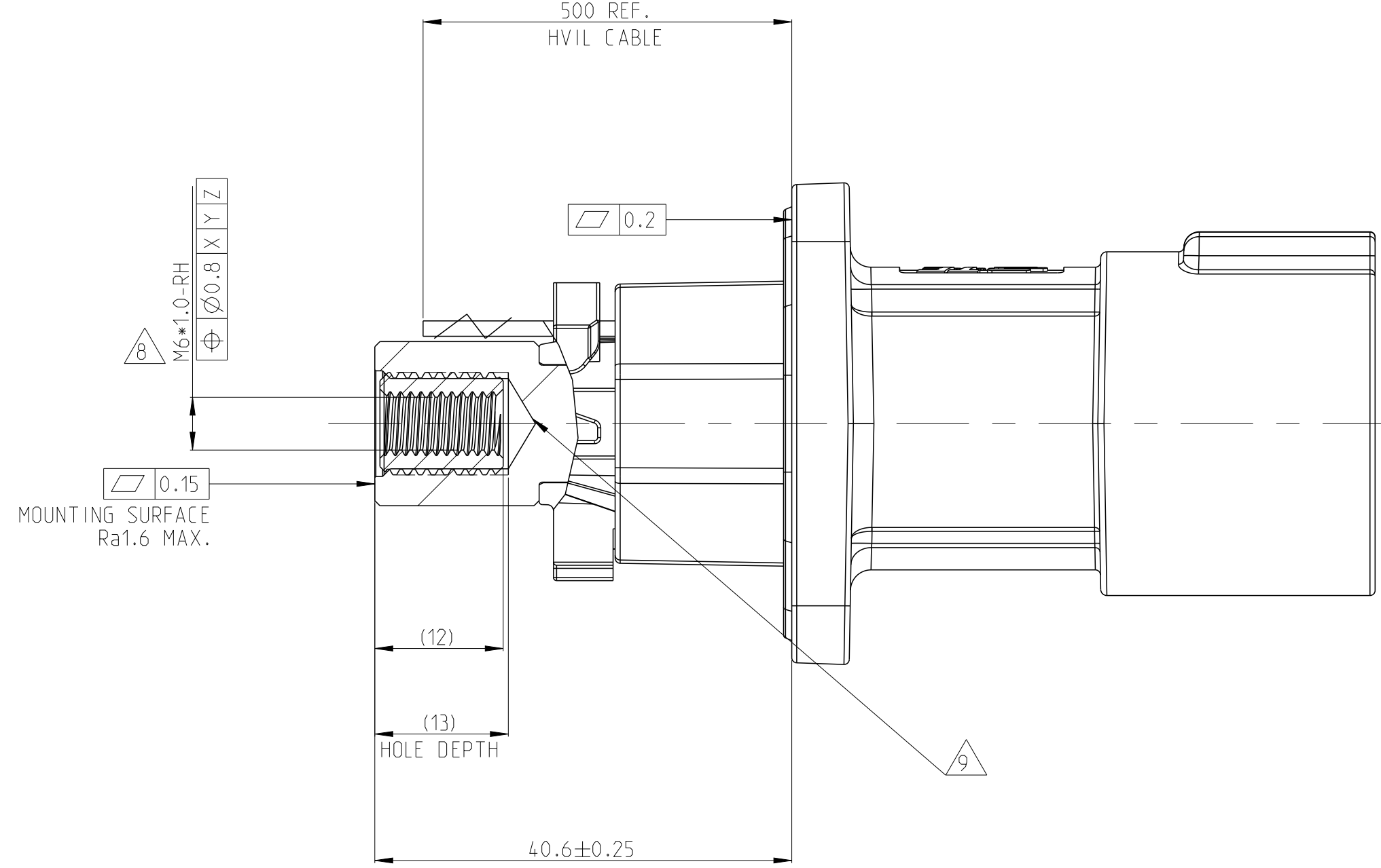
SECTION A-A
