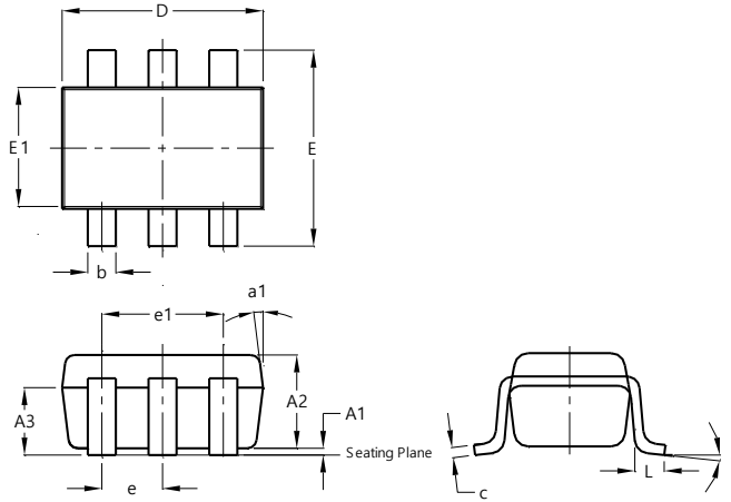
SOT28
