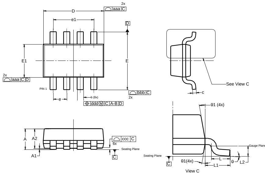
SO-8 (Standard)
