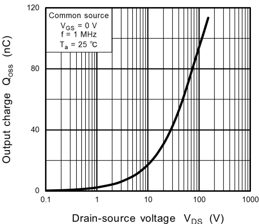
Fig. 8.12 Q_{oss} - V_{DS}
