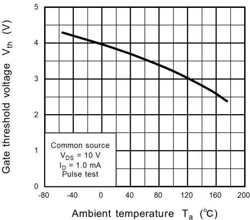
Fig. 8.8 V_{th} - T_a
