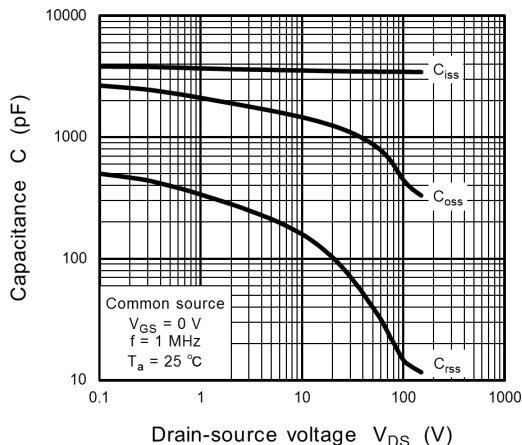
Fig. 8.11 Capacitance - V_{DS}
