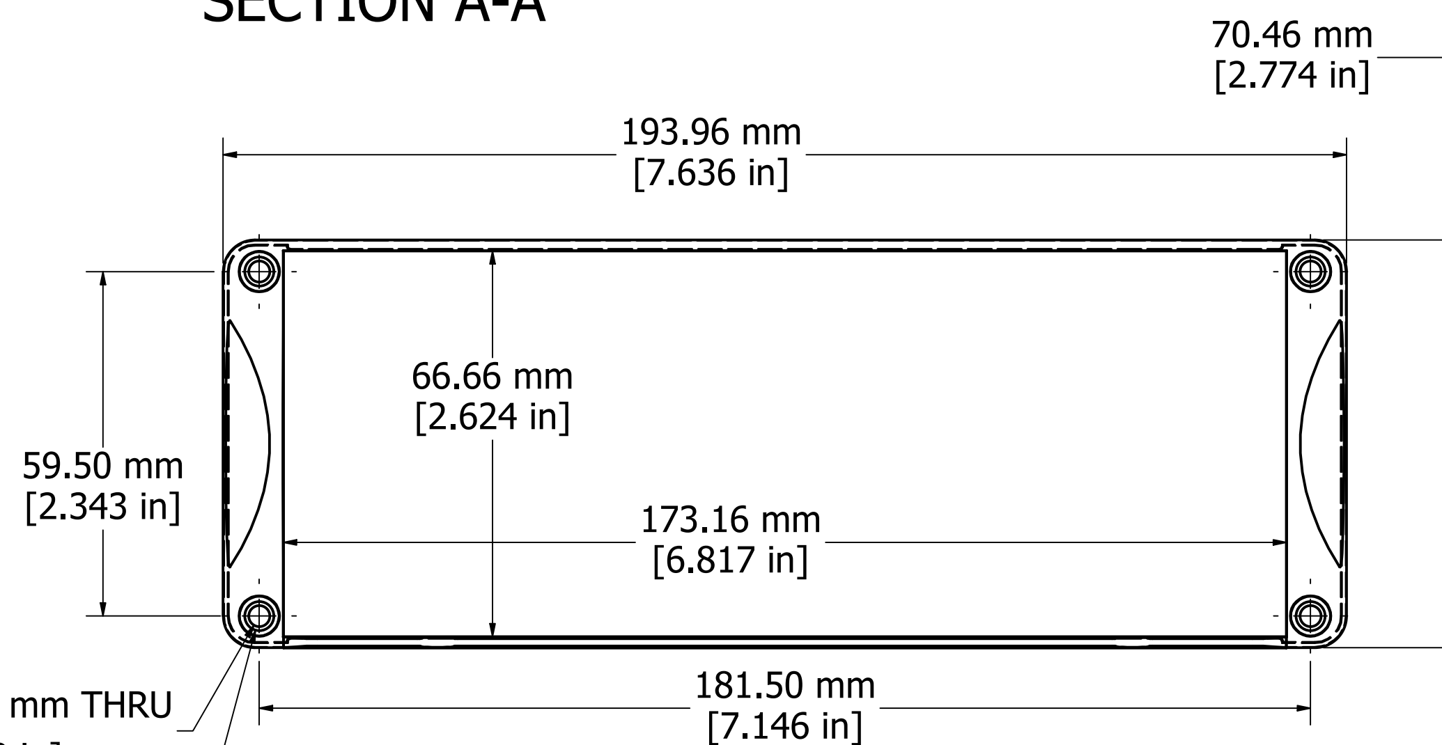
SECTION A-A
