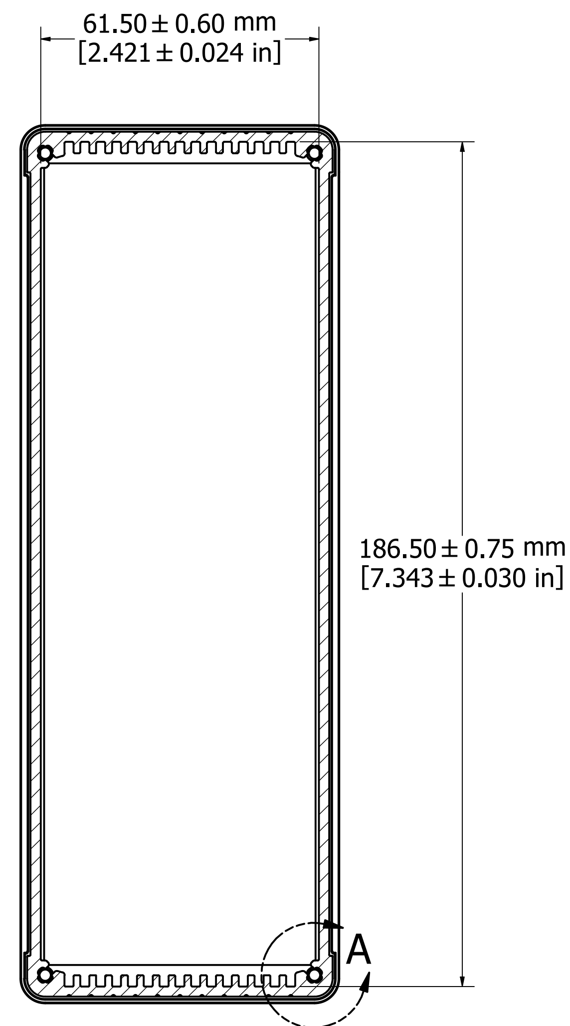
SECTION A-A
