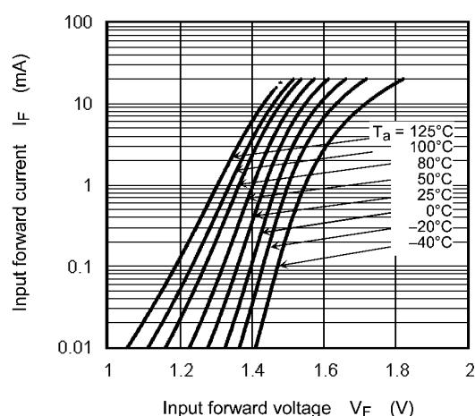
Fig. 13.2.1 I_F - V_F
