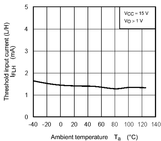
Fig. 13.2.4 I_{FLH} - T_a
