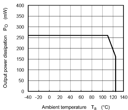
Fig. 13.2.3 P_O - T_a
