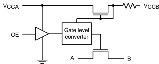
TC7SPB9306TU
