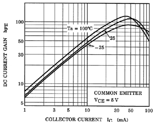
Fig. 10.13 RN1301 h_{FE} - I_C
