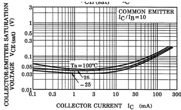
Fig. 8.3 V_{CE(sat)} - I_C
