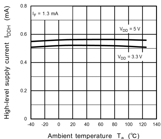
Fig. 12.2.7 I_{DDH} - T_a
