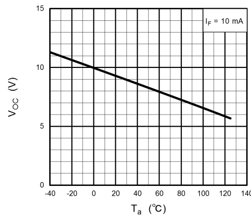
Fig. 12.6 V_{OC} - T_a
