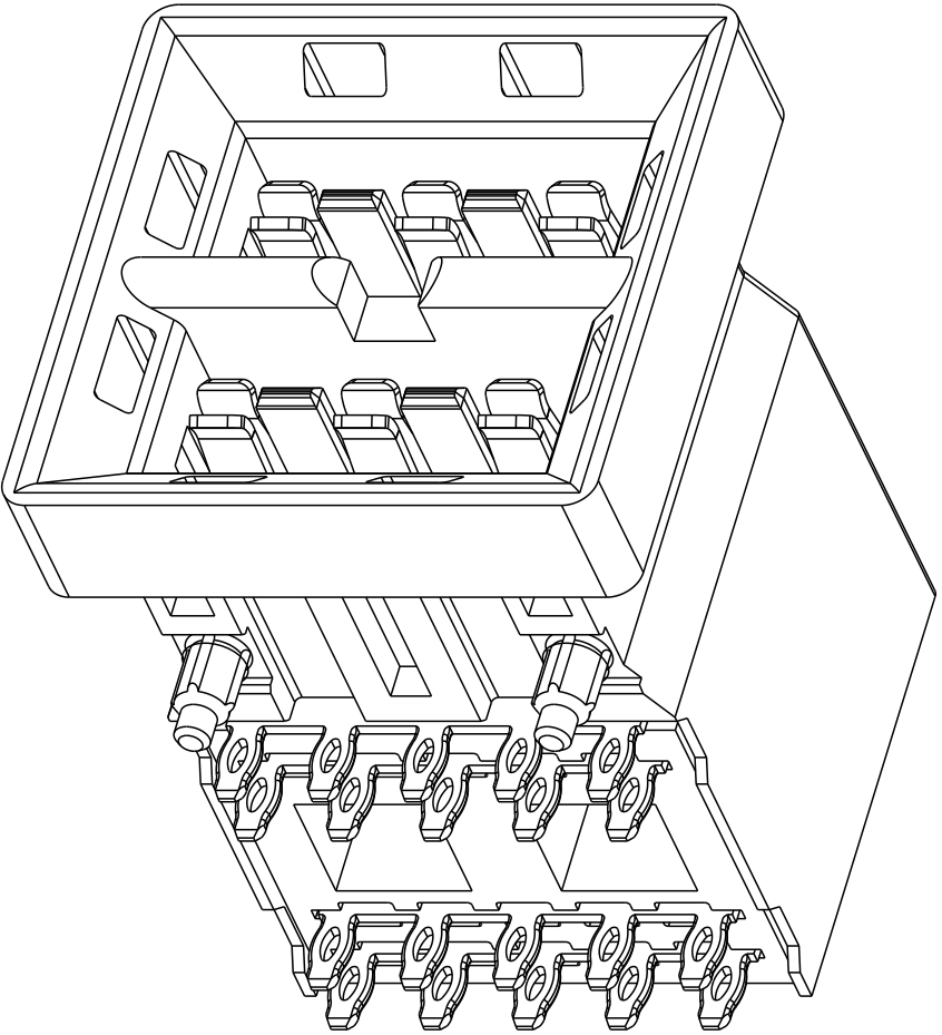
10132640-003LF SCALE 3:1
