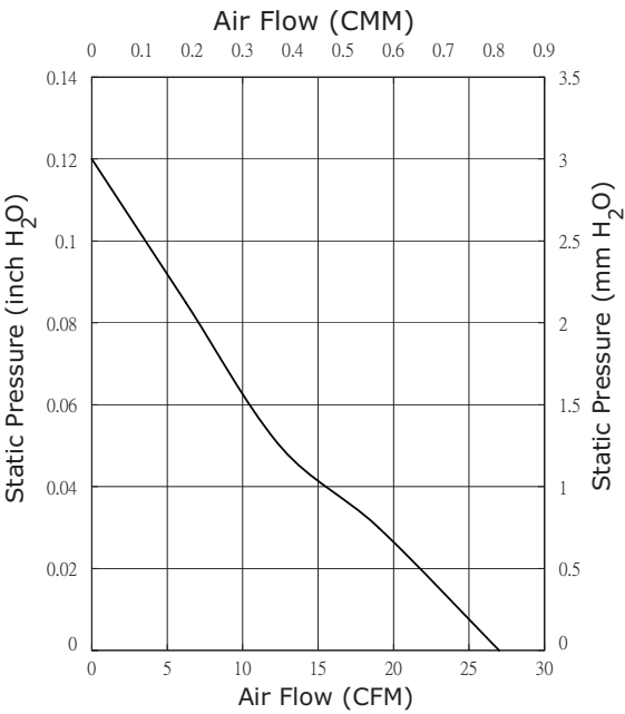
CFM-7020V-129-300
