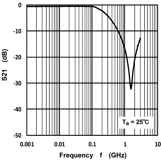
Fig. 10.1 S_{21} - f
