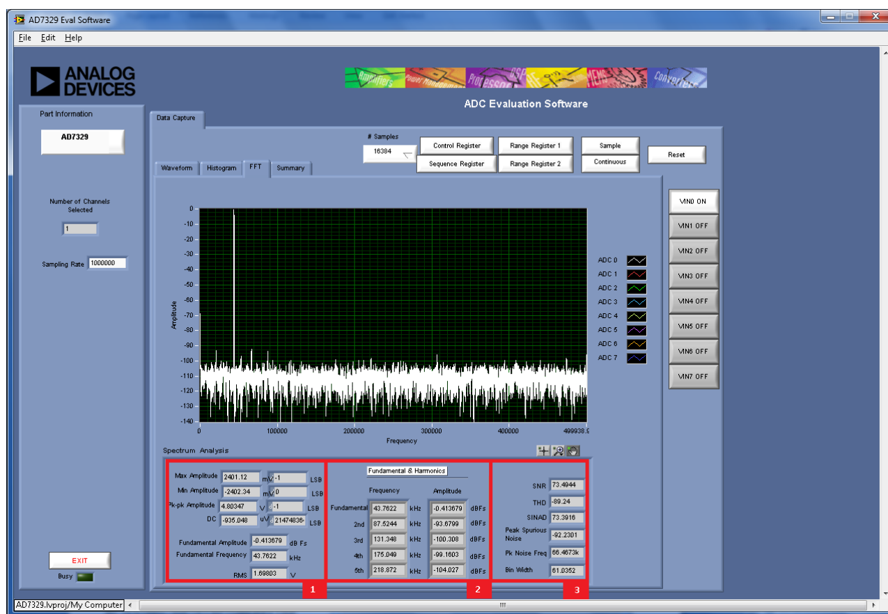
Figure 24. FFT Tab
