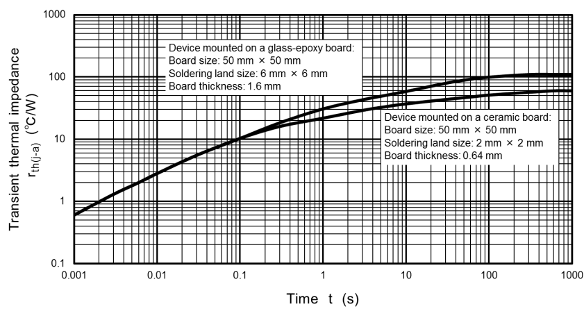
Fig. 10.7 r_{th(j-a)} - t
