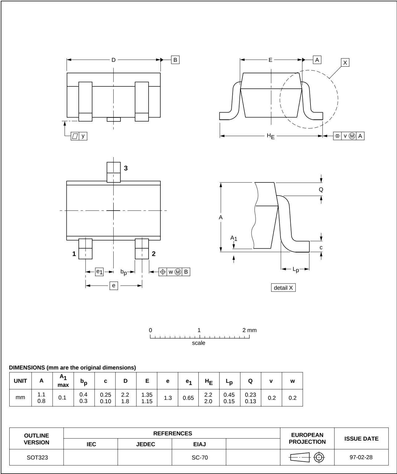
Fig 14. SOT323 (SC-70).
