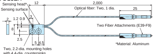
E32-D25Z E32-D25ZR
