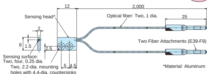
E32-D25XB
