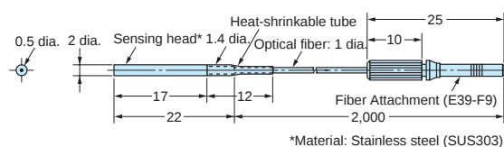
E32-T222 E32-T222R
