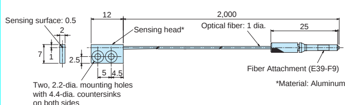
E32-TC200(F4) E32-TC200F(F4R)
