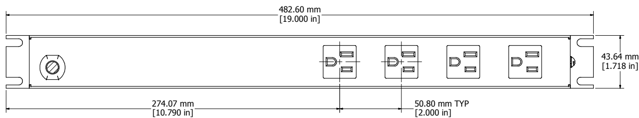
SECTION A-A
