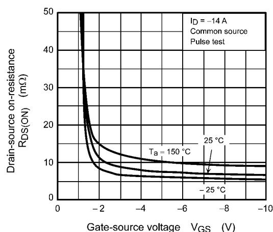
Fig. 8.4 R_{DS(ON)} - V_{GS}
