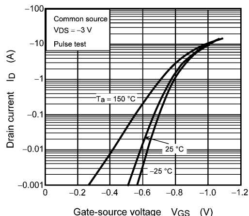
Fig. 8.2 I_D - V_{GS}
