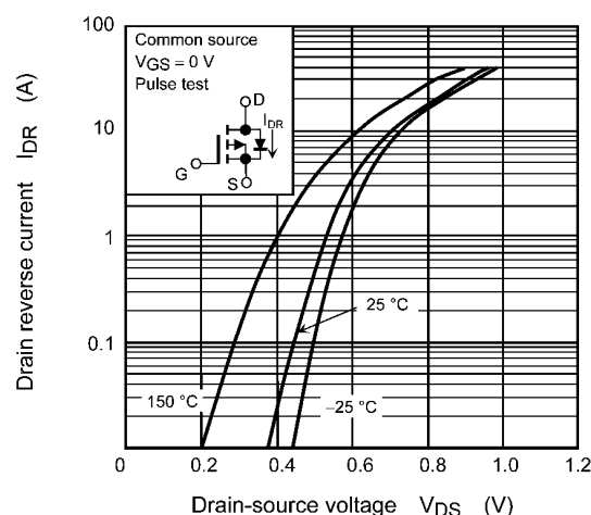
Fig. 8.12 I_{DR} - V_{DS}
