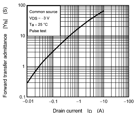
Fig. 8.8 |Y_{fs}| - I_D
