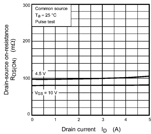
Fig. 8.4 R_{DS(ON)} - I_D
