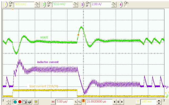
Figure 25. Load Transient, 5\text{ V}_{IN} , 0.9\text{ V}_{OUT} , 0.3\text{--}3\text{ A} , 100\text{ ns} Edge
