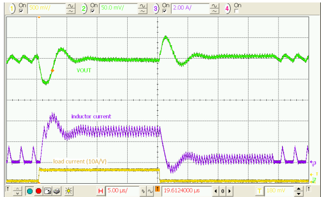
Figure 26. Load Transient, 3.6\text{ V}_{IN} , 1.2\text{ V}_{OUT} , 0.3\text{--}3\text{ A} , 100\text{ ns} Edge
