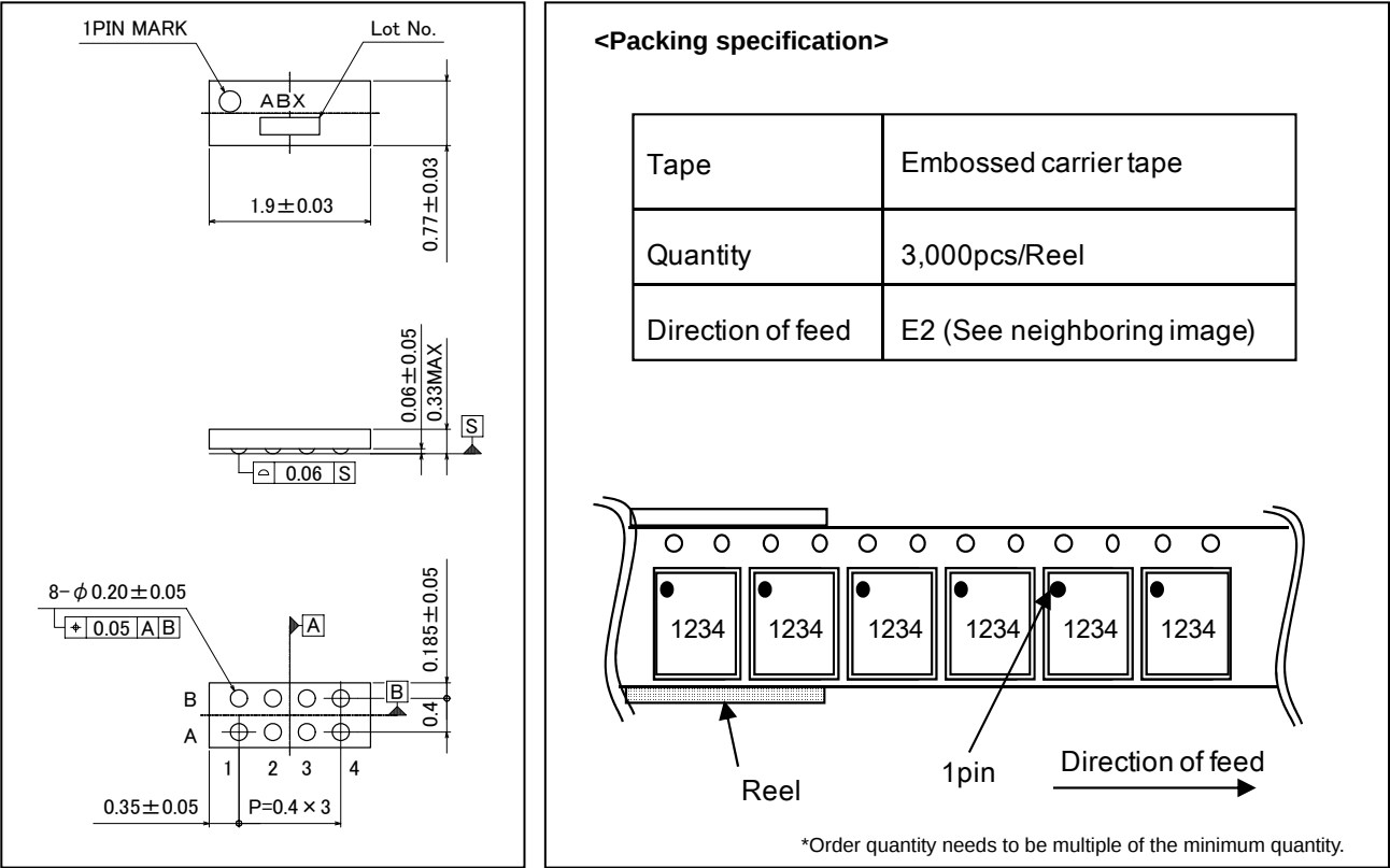
UCSP30L1 (BU64562GWZ)
