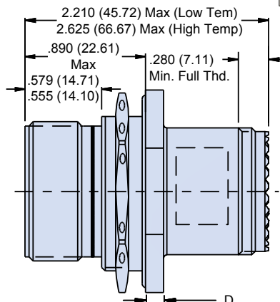
Jam Nut
