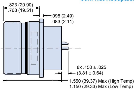
Jam Nut Receptacle
