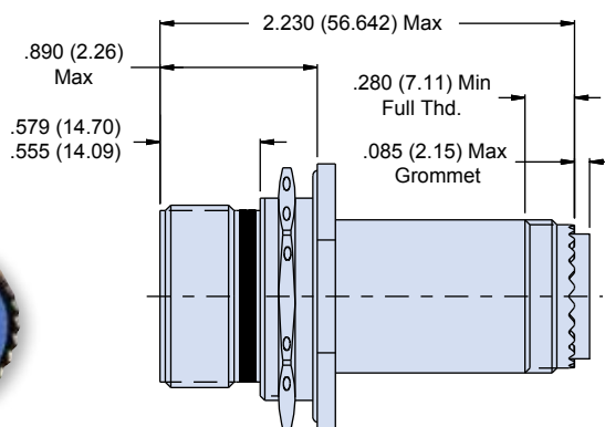
Jam Nut
