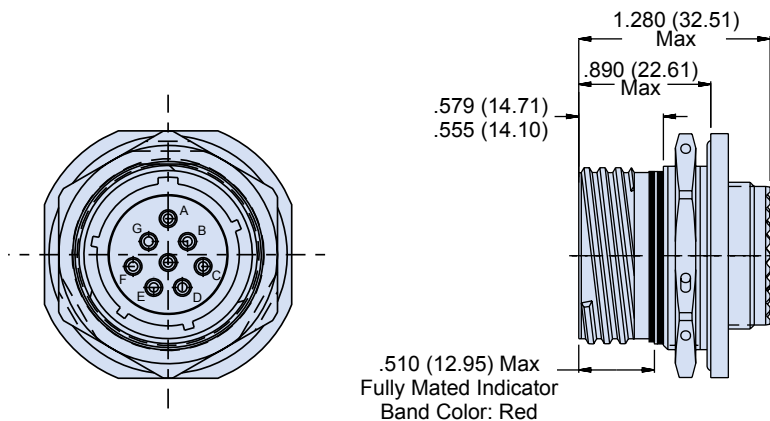
07 - Jam Nut Receptacle
