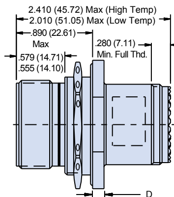
Jam Nut
