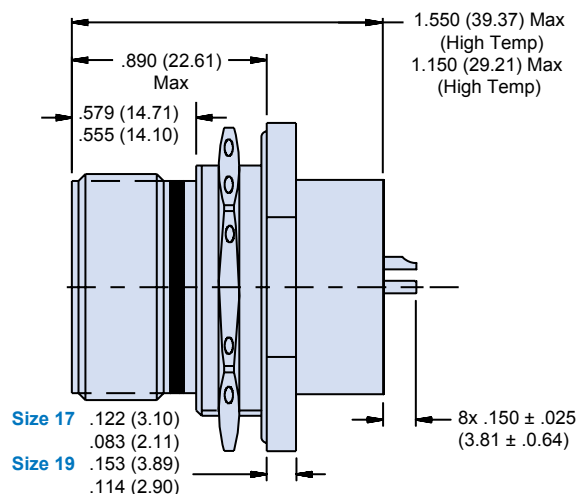
Jam Nut Receptacle
