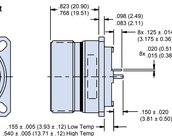
Jam Nut Receptacle
