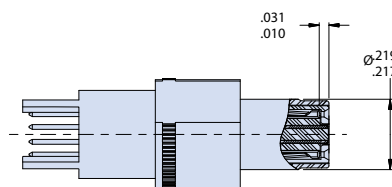
SIZE #8 EL OCHITO PIN, PC TAIL DETAIL
