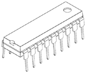
P-DIP18-300-2.54-001
