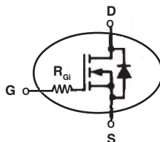
TO-268HV (IXTT..HV)
