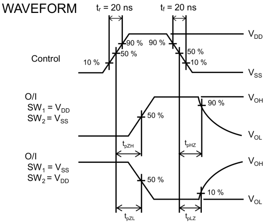
Fig. 11.1.2 t_{PZH} , t_{PHZ} , t_{PZL} , t_{PLZ}
