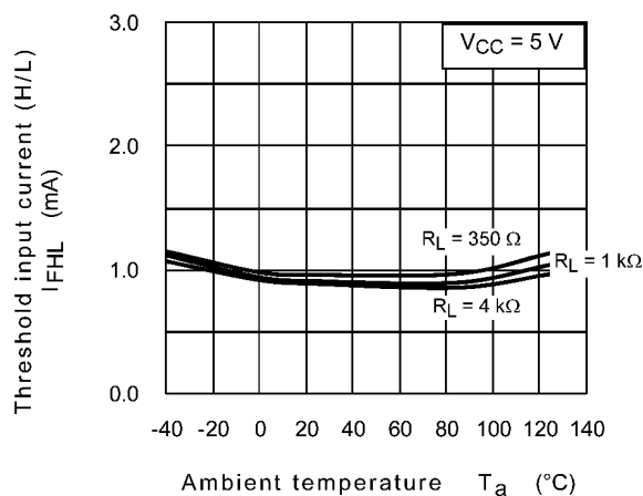
Fig. 12.2.7 I_{FHL} - T_a
