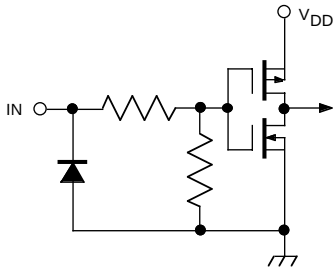
Dwg. EP-010-12
