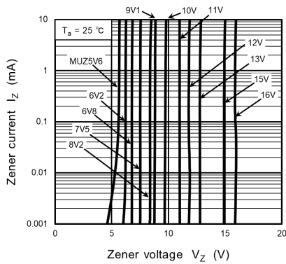
Fig. 10.1.1 I_Z - V_Z(1)
