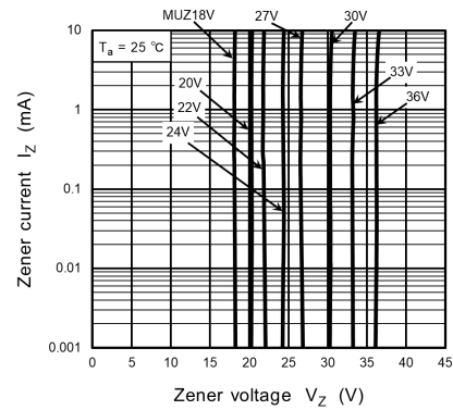
Fig. 10.1.2 I_Z - V_Z(2)
