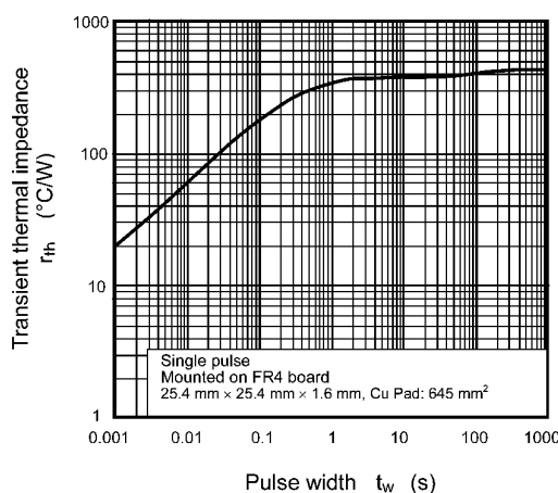
Fig. 7.11 r_{th} - t_w
