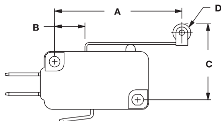
FIG. 2 Lever Roller
