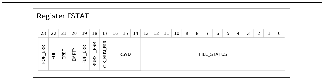
Figure 42 FSTAT Register
