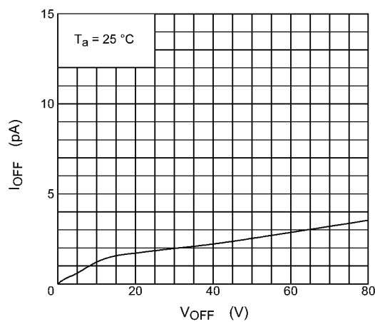
Fig. 12.9 I_{OFF} - V_{OFF}
