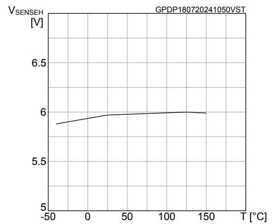
Figure 26. V_{\text{senseh}} vs T_C
