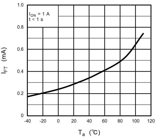
Fig. 14.1.6 I_{FT} - T_a
