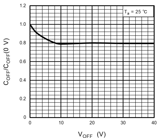
Fig. 14.1.11 C_{OFF} - V_{OFF}
