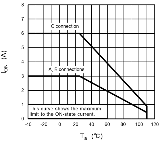
Fig. 14.1.2 I_{ON} - T_a
