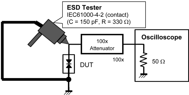
Fig. 6.1.3 IEC61000-4-2 (Contact)
