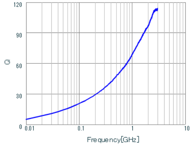
LQW18AN3N6C00 Q.
