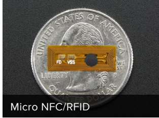
13.56MHz RFID/NFC tag
