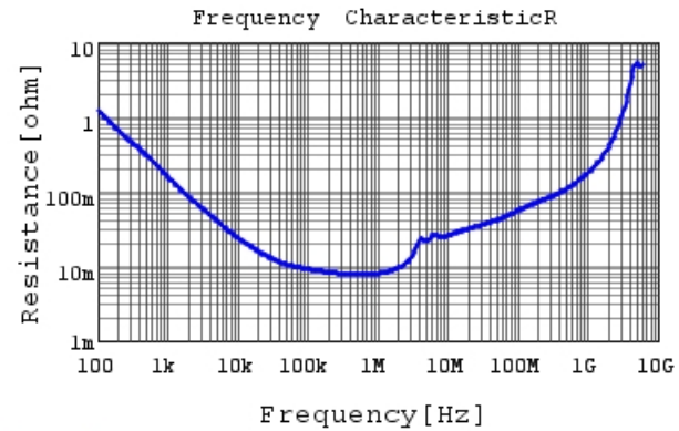
GRJ31CR71H475ME11 R DCOV,25degC
