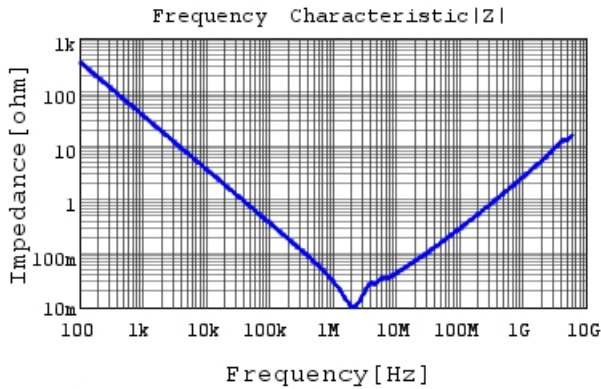
GRJ31CR71H475ME11 |Z| DCOV,25degC
